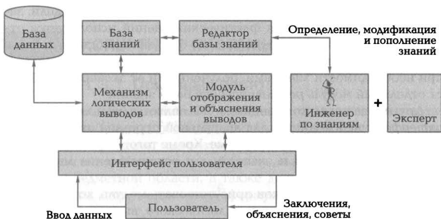
Рис. 11.8. Структура экспертной системы
