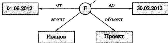
Рис. 11.5. Представление события
