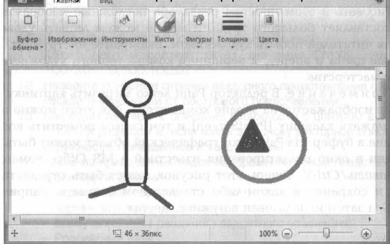
Рис. 4.4. Редактор Paint
